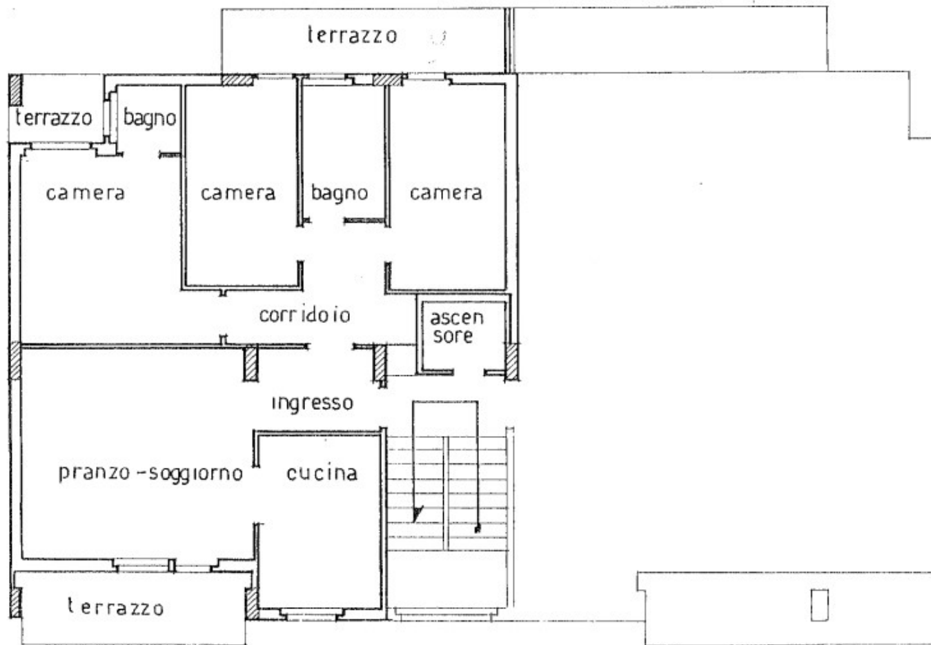
PÍANO TERZO
